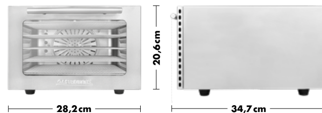
Ventilator und Heizelement an der Rückseite – ermöglicht absolut gleichmäßiges Trocknen für beste Ergebnisse
